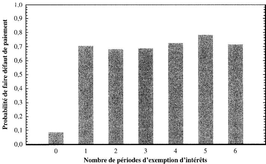
GRAPHIQUE 3 COHORTE 1990-1991 PROBABILITÉ DE FAIRE DÉFAUT DE PAIEMENT CONDITIONNEL AU NOMBRE DE PÉRIODES D'EXEMPTION D'INTÉRÊTS
