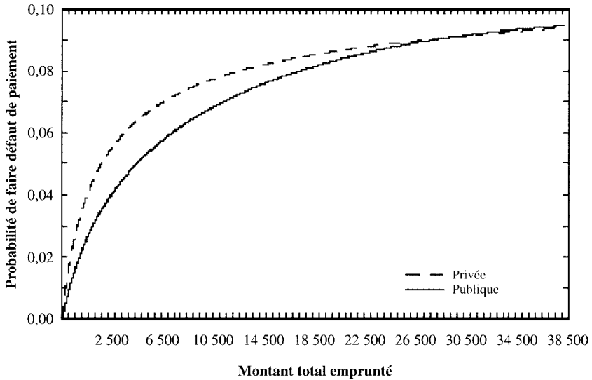
GRAPHIQUE 4 COHORTE 1990-1991 PROBABILITÉ DE FAIRE DÉFAUT DE PAIEMENT RELATIVEMENT AU MONTANT EMPRUNTÉ PAR TYPE D'INSTITUTION
